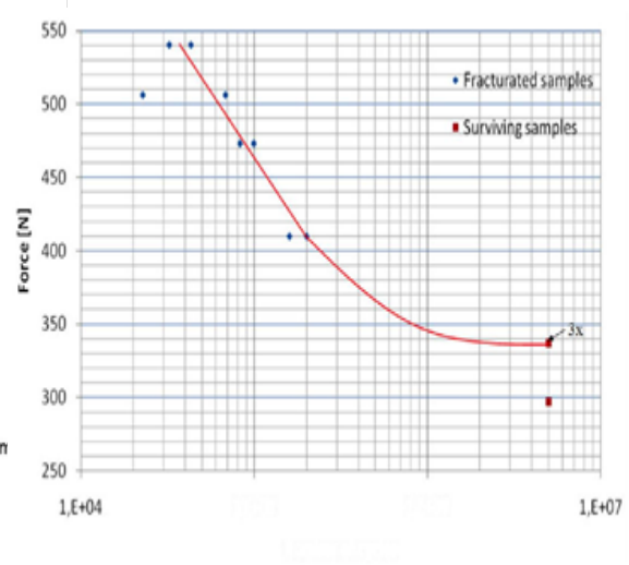
Fig.5 Curba Wöhler a Sistemului B
