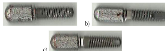
Fig.1 Specimene ce au rezistat la testul de oboseală (5mil. cicluri) a) Sistemul A; b) Sistemul B; c) Sistemul C
