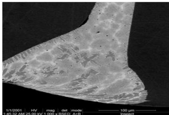
Fig. 8. Secțiune transversală prin îmbinarea de colt (proba T) (1000x).
