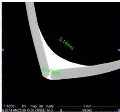
Fig. 7. Secțiune transversală prin îmbinarea de colt (proba T) (50x).
