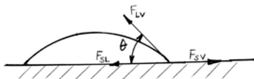
Fig.1. Sistemul de forte care acționează asupra metalului topit la brazare:
